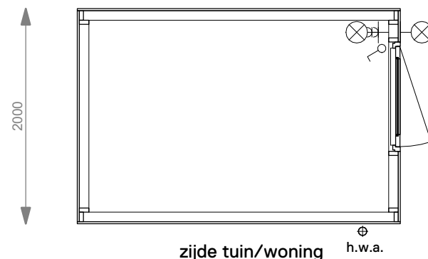
Begane grond
